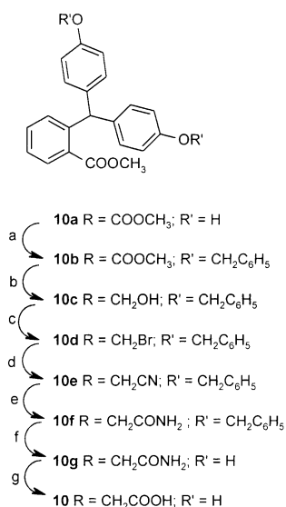
Scheme 2. (a) C 6 H 5 CH 2 Br, K 2 CO 3 ; (b) LiAlH 4 ; (c) PBr 3 ; (d) NaCN; (e) NaCN; (e) NaOH; (f) H 2 /Pd-C; (g) NaOH.
